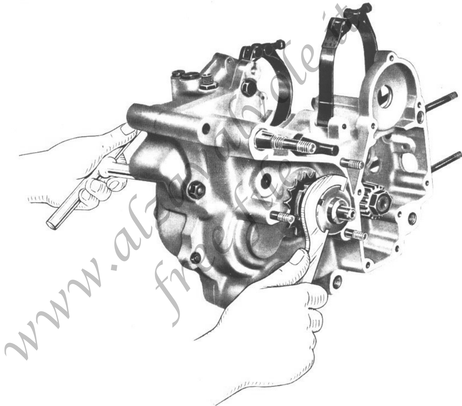
Fig. 11 - Come si leva il manicotto dentato per la messa in moto
