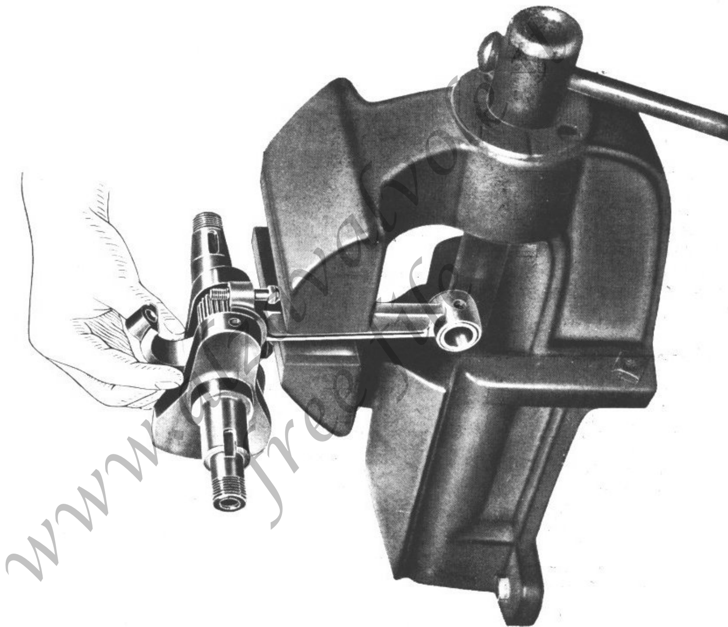
Fig. 20 - Come viene eseguito il montaggio della biella e degli aghi sull'albero a gomito 51
